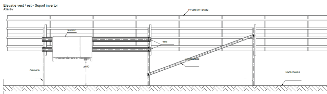
Figura 3. Desen indicativ – Detalii structură – soluție pentru structura de montare a invertoarelor
